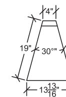
KR19-F30
