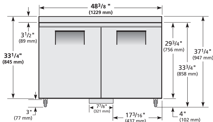
ELEVATION
